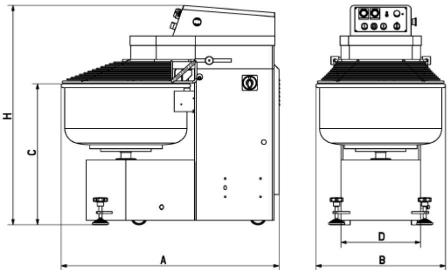
Dimensioni ingombro (cm)-Overall dimensions-Dimensions d'encombrement-Abmessungen-Dimensiones en el espacio
